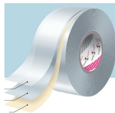
ochranná fólie hliníková fólie polyakrylátové lepidlo
